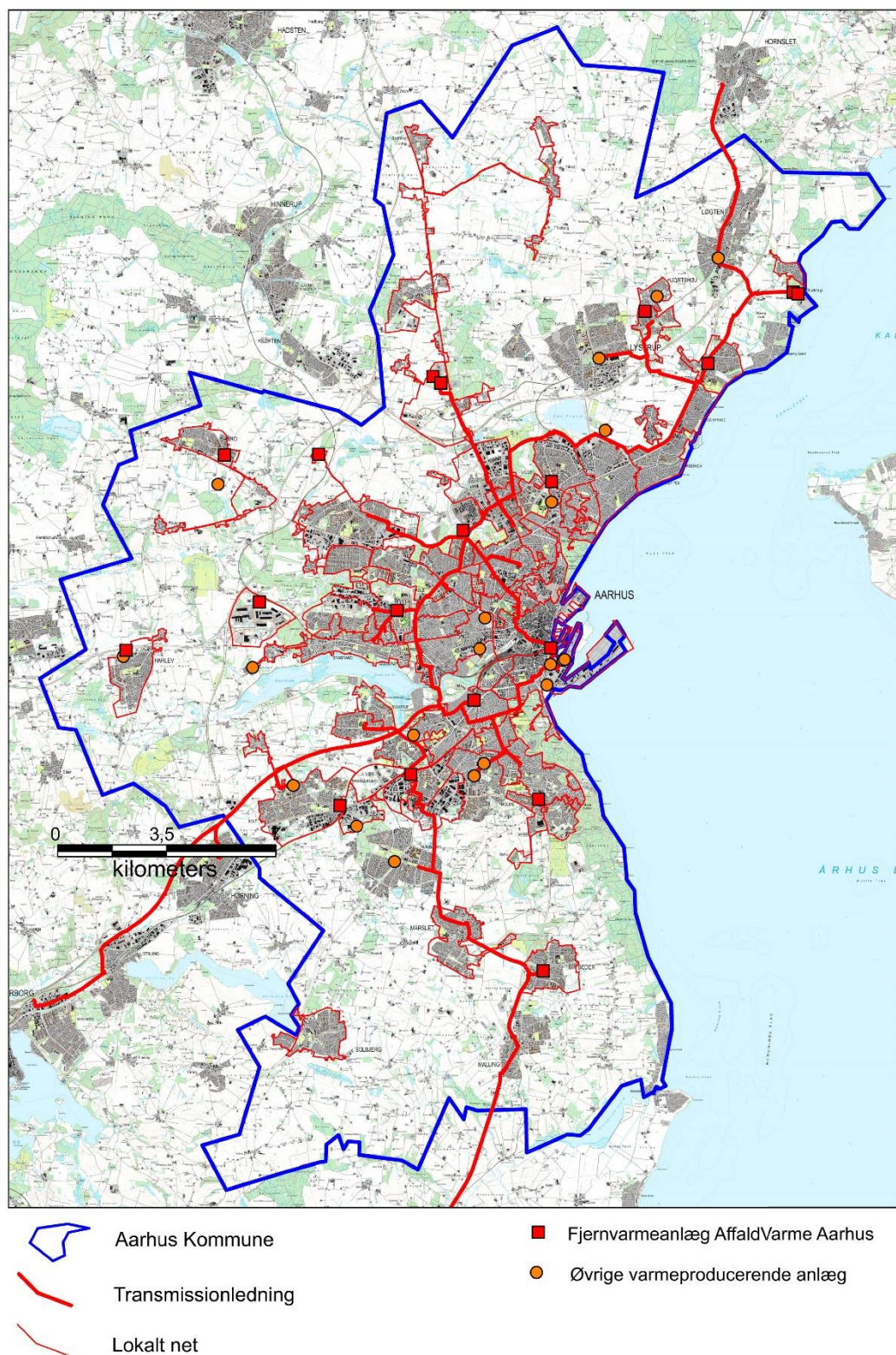
Figur 2.1. Kort over distributionsnet og varmeproducerende anlæg.
