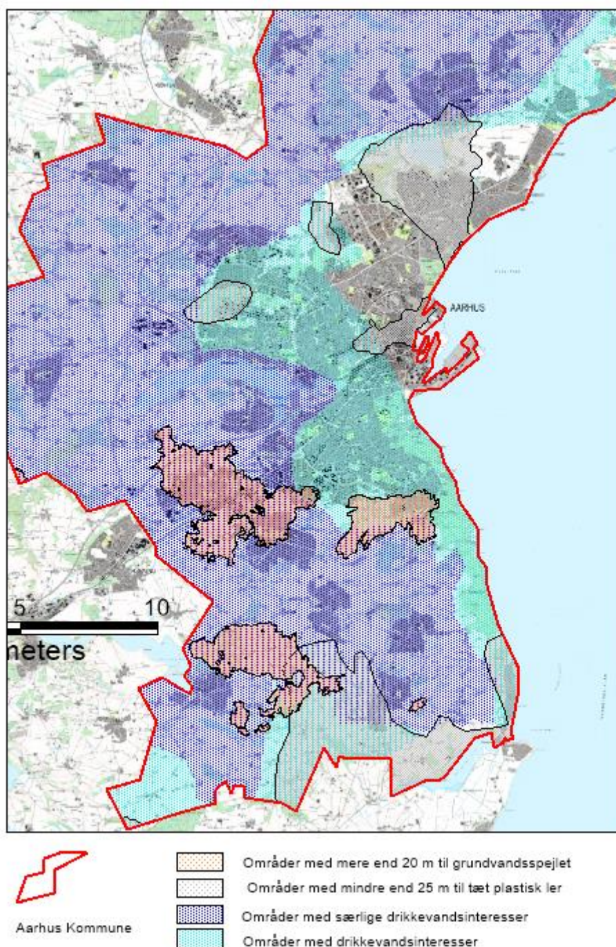
Figur 3.4. Områder potentielt egnet til BTES.
